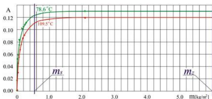
Rys. 1. Wykres pochłaniania promieniowania cieplnego przez dwutlenek węgla, uwzględniający masę nasycenia m_s i masę CO 2 w atmosferze ziemskiej m_z
