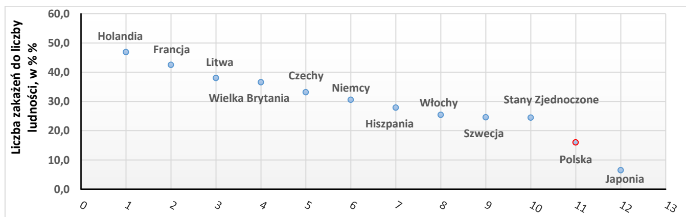
Rys. 1. Zestawienie liczby zakażeń na Covid-19 do liczby mieszkańców, w wybranych krajach, wyrażone w %%
