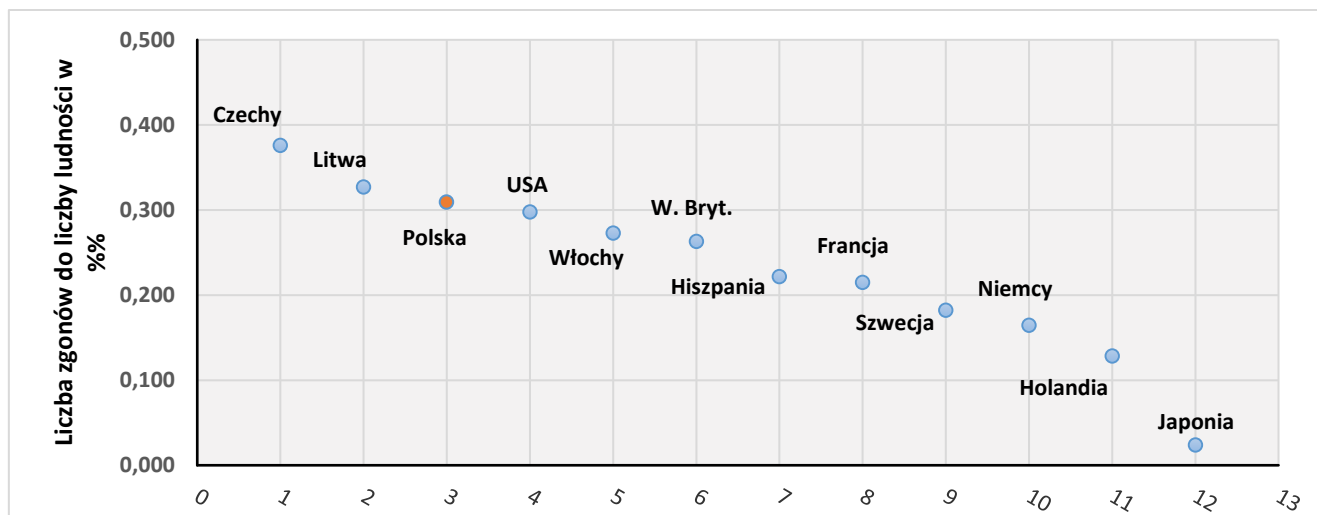
Rys. 2. Zestawienie liczby zgonów z powodu Covid-19 do liczby mieszkańców, w wybranych krajach, wyrażone w %%
